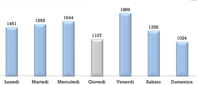
Andamento dei flussi veicolari settimanali 6/03/2017 - 12/03/2017
