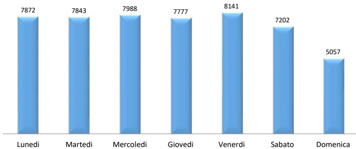
Andamento dei flussi veicolari settimanali 6/03/2017 - 12/03/2017
