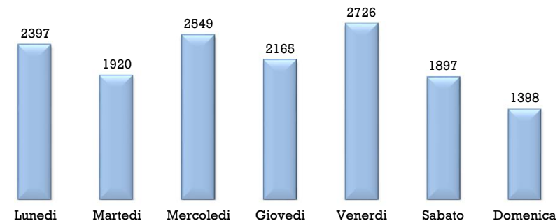
Andamento dei flussi veicolari settimanali 6/03/2017 - 12/03/2017
