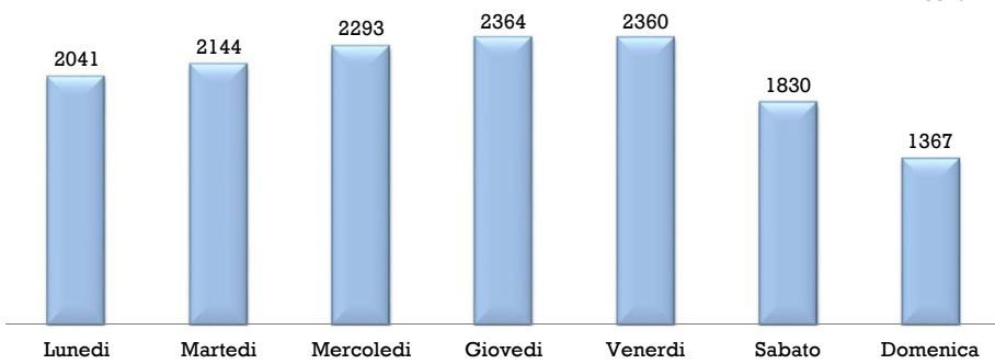
Andamento dei flussi veicolari settimanali 6/03/2017 - 12/03/2017
