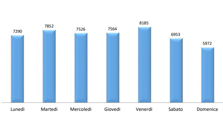
Andamento dei flussi veicolari settimanali 6/03/2017 - 12/03/2017
